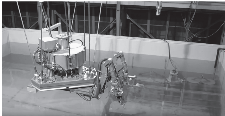
Vienas iš robotų, dirbančių Fukušimos reaktoriaus bloke.
